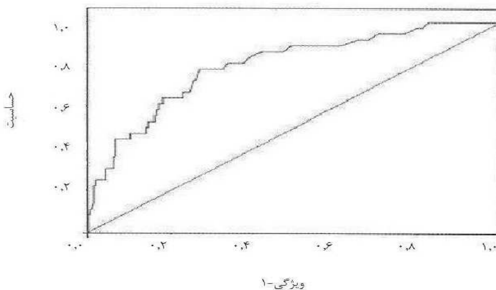
شکل ۱: آنالیز منحنی ROC برای احتمال مرگ محاسبه شده بر اساس شاخص PIM2
