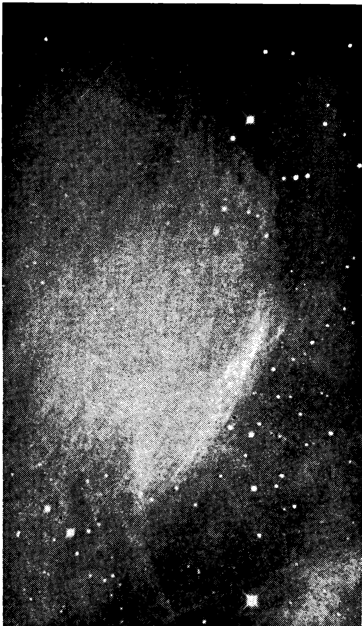
شکل ۷۹- چنین نظر میرسد که این ابزار نوری در بینه آسمان آبی دستخوش بادگشته است . این عکس حوالی یکی از ستاره گان بر زمین است که با عدسی ۵ پایی برداشته شده ( عکس در سال ۱۹۰۹ در رصدخانه منت ویلسون در مدت ۵ ساعت گرفته شده )
