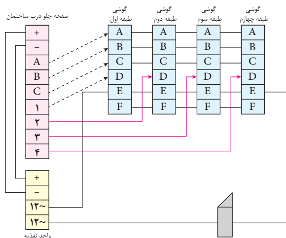
شکل ۲۱ - سیم کشی آیفون تصویری
