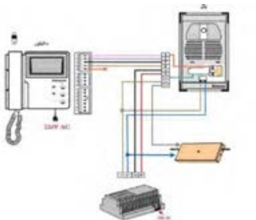
شکل ۲۷ - سیم‌بندی کامل آیفون تصویری برای یک واحد
