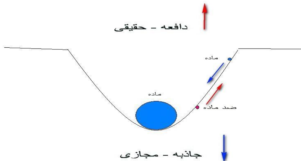
نمودار فضا زمان ماده و ضد ماده
