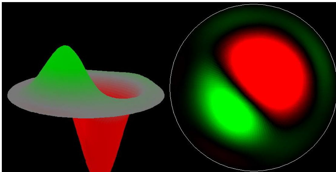
نمودار فضا زمان ماده و ضد ماده
