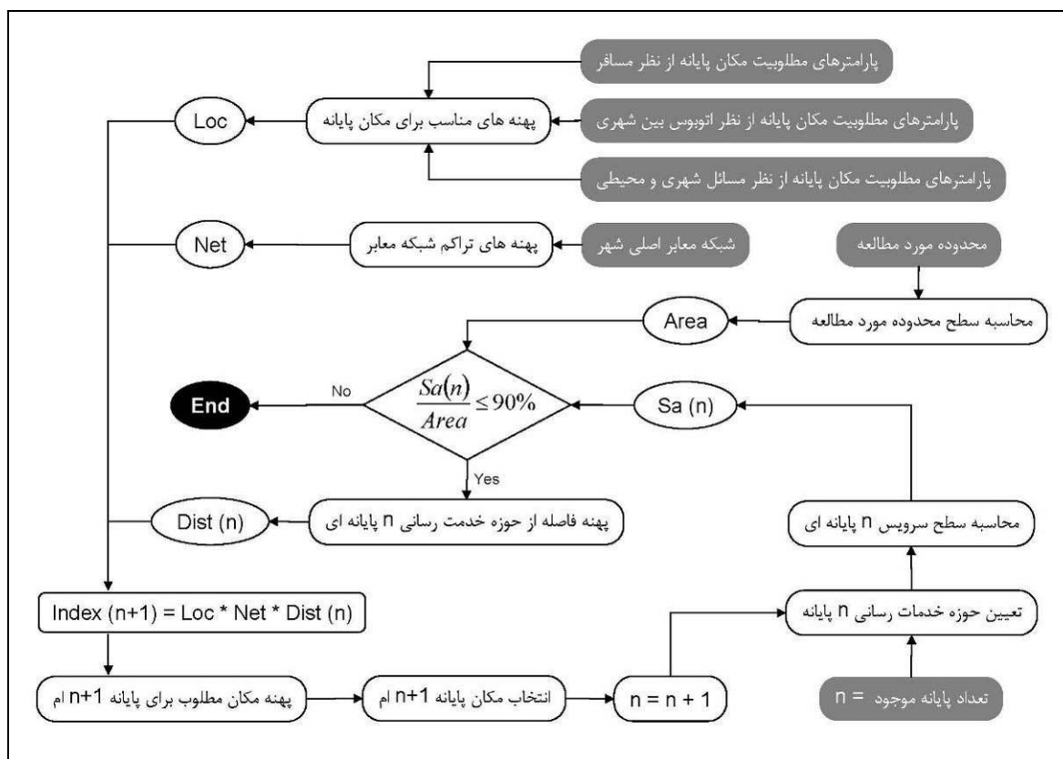
شکل ۴-۵: الگوریتم مکان‌یابی پایانه‌های (متمرکز و نیمه متمرکز).
