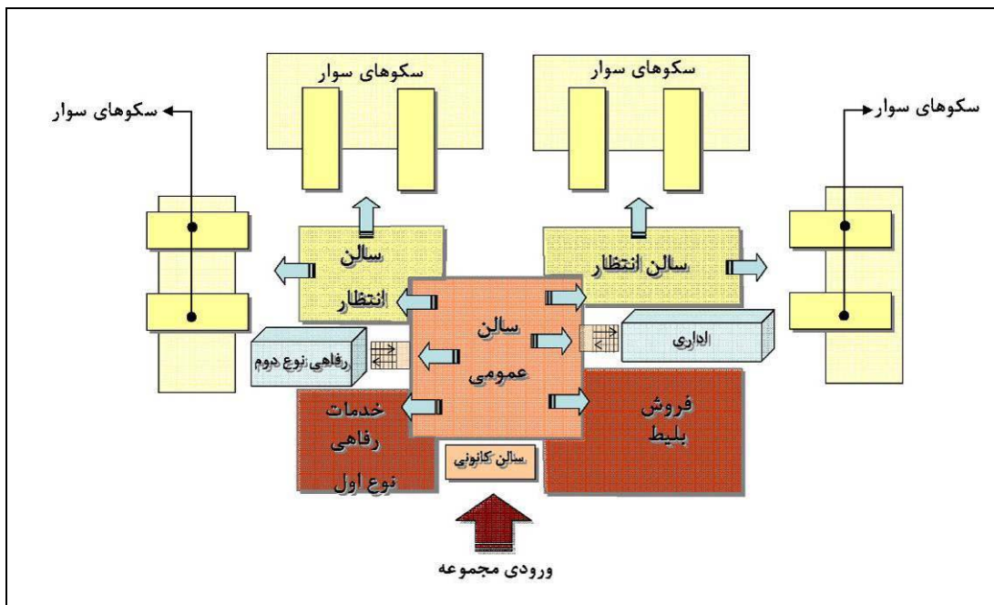
شکل ۲-۵: دیاگرام ارتباطی فضاها و بخشهای داخلی کالبد پایانه متمرکز
