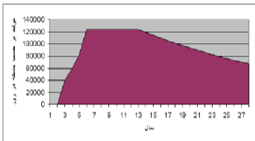
نمودار ۳- نحوه‌ی توزیع تولید میادین سیری A و E
