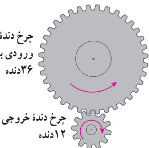
شکل ۱۶ - به ازای هر بار چرخش چرخ‌دنده بزرگ چرخ‌دنده کوچک سه بار می‌چرخد.
