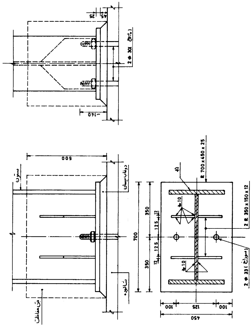
شکل ۱۲-۲۸ کف ستون نوع اقتباس از کارخانه ماشین سازی تبریز [۱۴]
