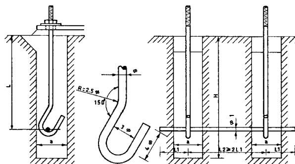
شکل ۱۲-۱۸ پیچ مهراری با قلاب انتهایی و رکاب [۱۴]
