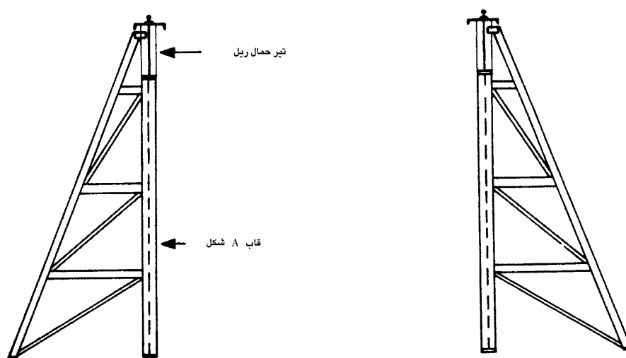
شکل ۹-۴-الف تکیه‌گاه‌های ریل داخل ساختمان برای جرثقیل‌های بالانشین [۱۶]
