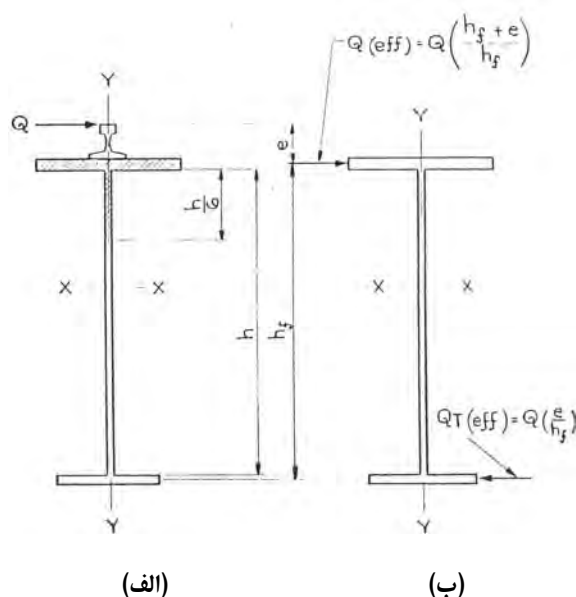
شکل ۶-۱ سطح مقطع موثر در محاسبه تنش ناشی از بار جانبی و بار جانبی اصلاح شده [۱۵]
