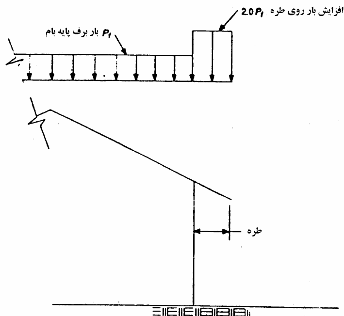
شکل ۲-۳ بار اضافی روی بخش طره بام [۱۶]
