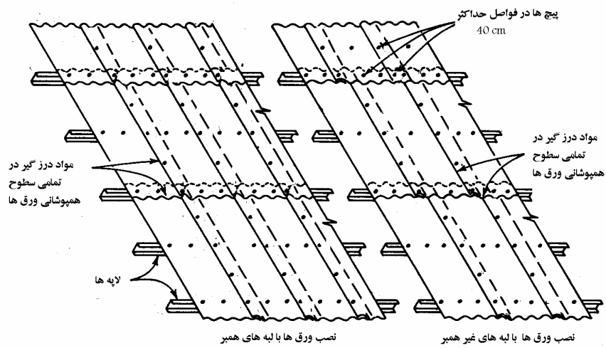
شکل ۷-۴-الف نصب ورق ها با لبه های غیر همبر و همبر
