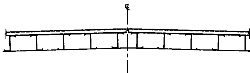
شکل ۸-۷ جهت‌گیری لاپه‌های در سقف‌های با شیب کم [۱۷]
