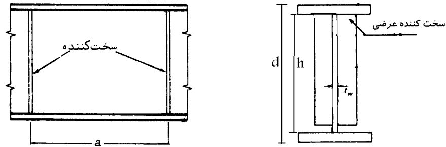
شکل ۳-۴ مقاطع تقویت‌کننده عرضی
