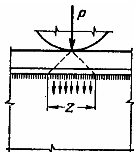
شکل ۵-۶ توزیع بار متمرکز چرخ جرثقیل در ناحیه اتصال جان و بال تیر [۳۵]
