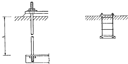
شکل ۱۲-۲۱ پیچ مهاري با نبشي مهاري [۱۴]
