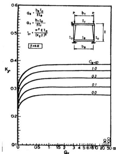
شکل D1-8 ضریب طول مؤثر برای ستون‌های با مقطع متغیر حرکت جانبی مقید \gamma=4 [۷]
