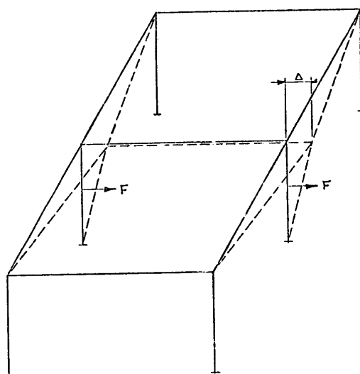
شکل ۹-۵ مهاربندی سقف [۲]
