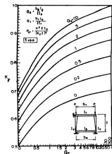
شکل D1-۲ ضریب طول مؤثر برای ستون‌های
