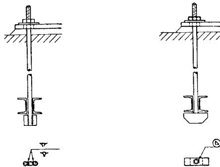
شکل ۱۲-۲۲ پیچ مهاري کلنگي [۱۴]
