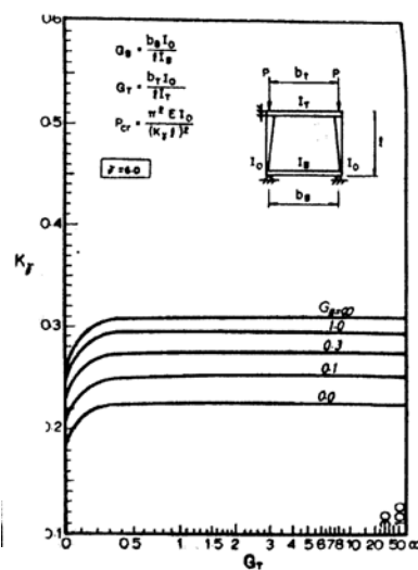
شکل D1-9 ضریب طول مؤثر برای ستون‌های با مقطع متغیر حرکت جانبی مقید \gamma=6 [۷]
