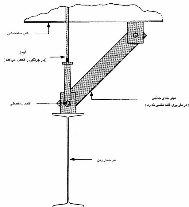
شکل ۴-۱۱-ب تعلیق انعطاف‌پذیر برای جرثقیل‌های آویخته و تک ریل [۱۶]
