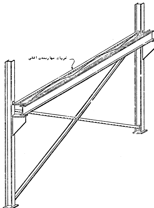
شکل ۶-۳ مهاربندی تیر باربر ریل [۲]
