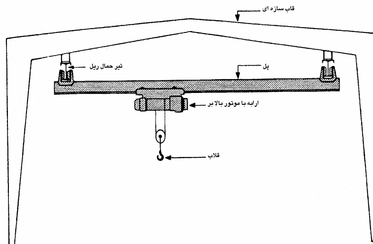
شکل ۳-۴ جرثقیل پل‌دار آویخته [۱۶]
