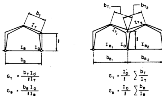
شکل D1-۱ تحلیل ضریب طول مؤثر در ستون‌های با مقطع متغیر [۷]
