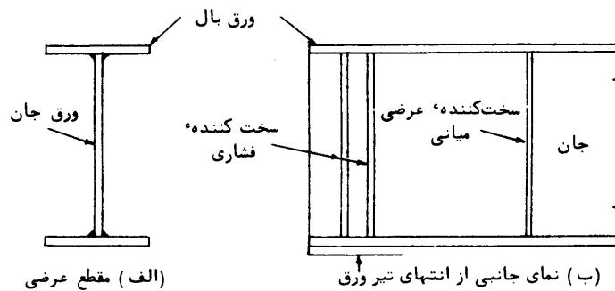
شکل ۳-۵ تیر ورق
