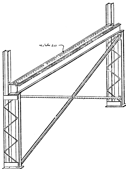
شکل ۶-۴ مهاربندی تیر باربر ریل [۲]
