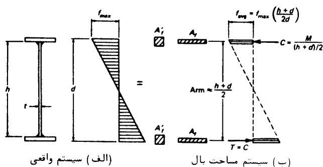
شکل ۹-۳ سطح مقطع بال برای برقراری رابطه مساحت بال [۸]
