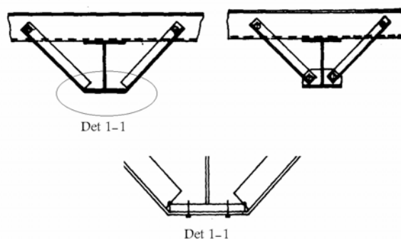
شکل ۷ مهاربندی بال فشاری [۳]
