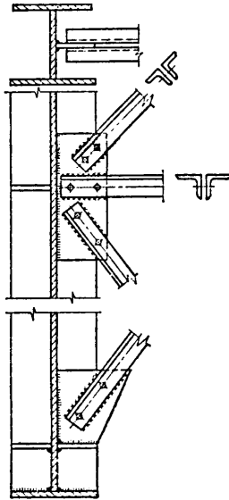
شکل ۹-۹ طراحی مهارهای قائم و اتصال‌شان به ستون‌ها [۲]
