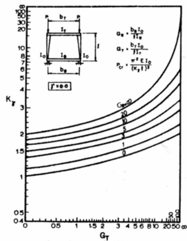
شکل D1-10 ضریب طول مؤثر برای ستون‌های با
