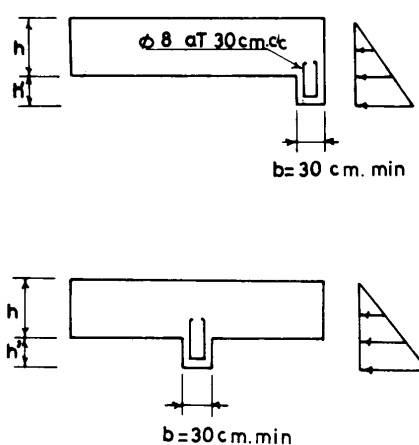
شکل ۱۲-۲ استفاده از برشگیر در زیر پی
