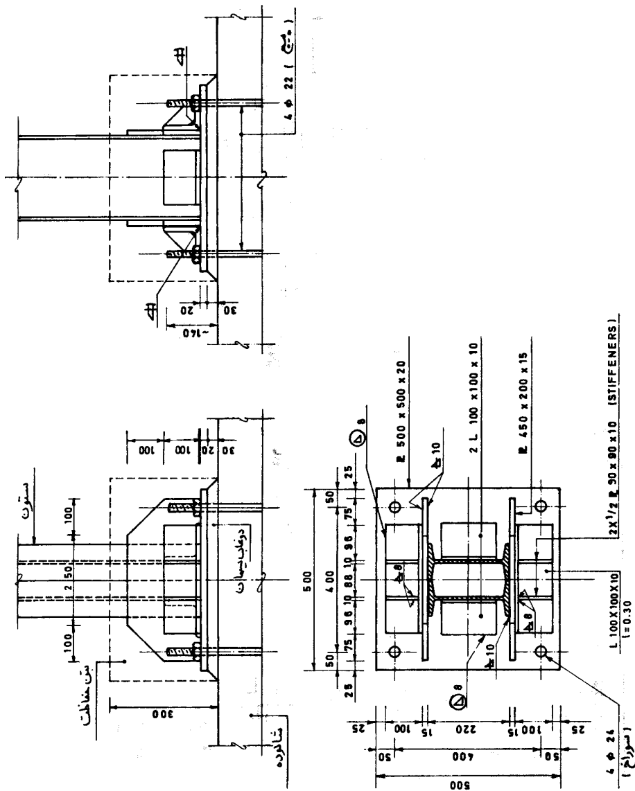
شکل ۱۲- ۲۷ کف ستون نوع اقتباس از توسعه کارخانه گچ تهران [۱۴]
