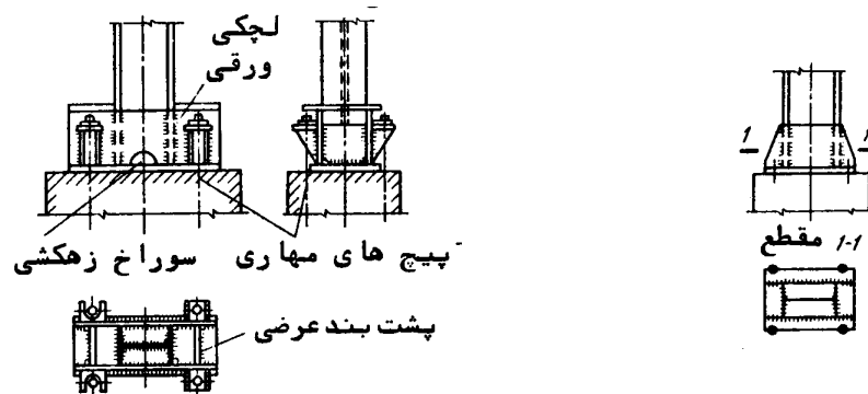
شکل ۱۲-۸ استفاده از قطعات ورق و یا لچکی [۱۴]
