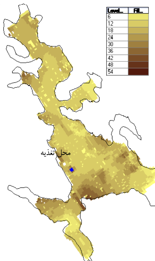
پراکندگی نیترات از منبع تغذیه
