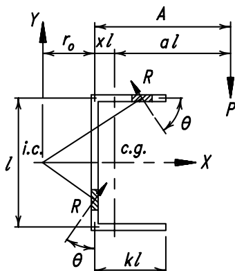
Fig. C-A-J2.1. Weld element nomenclature.
