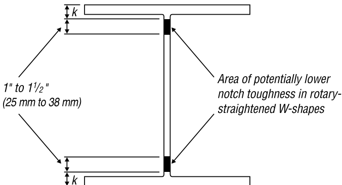
Fig. C-A3.2. "k-area."
